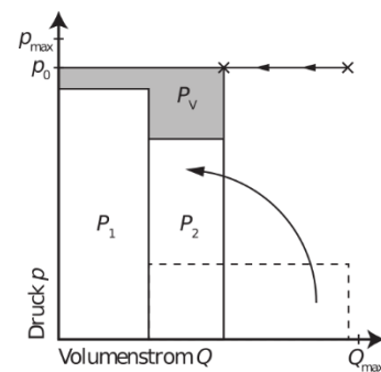
Abb: pQ-Diagramm Regenerations-Modus
